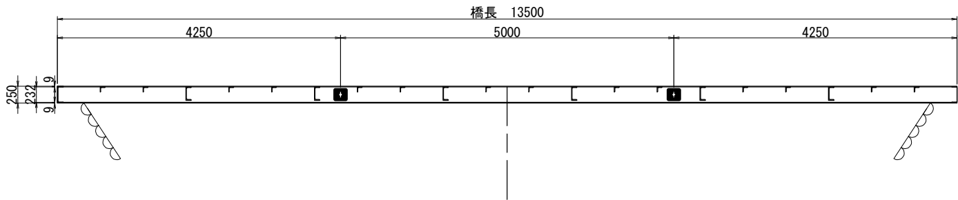
立面図
